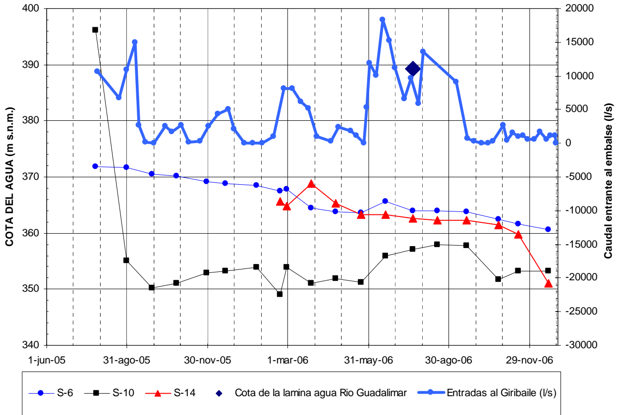
FIGURA 6 a.- ACUÍFERO CARBONATADO DE UBEDA. EVOLUCIÓN PIEZOMÉTRICA 2005-2006 (Entorno piezómetro S-10)
