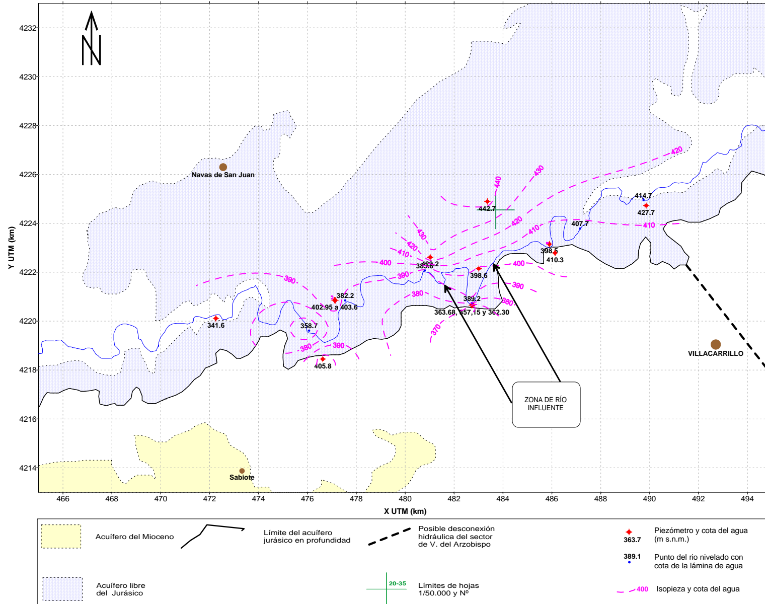
FIGURA 3.- COTAS DEL AGUA EN EL ENTORNO DEL RIO GUADALIMAR E ISOPIEZAS ORIENTATIVAS (16-07-2006)
