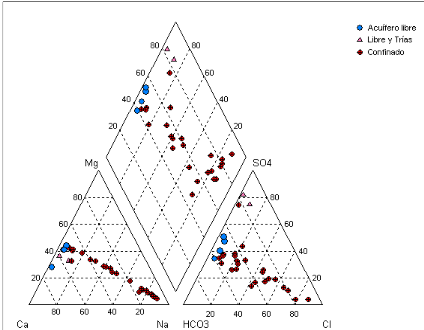
Figura 16.- Diagrama de Piper de la Campaña de muestreo de Julio de 2005
