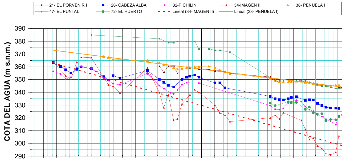
FIGURA 9.- ACUÍFERO CARBONATADO DE UBEDA. EVOLUCIÓN PIEZOMÉTRICA 2001-2006 (Sondeos más representativos del acuífero confinado)
