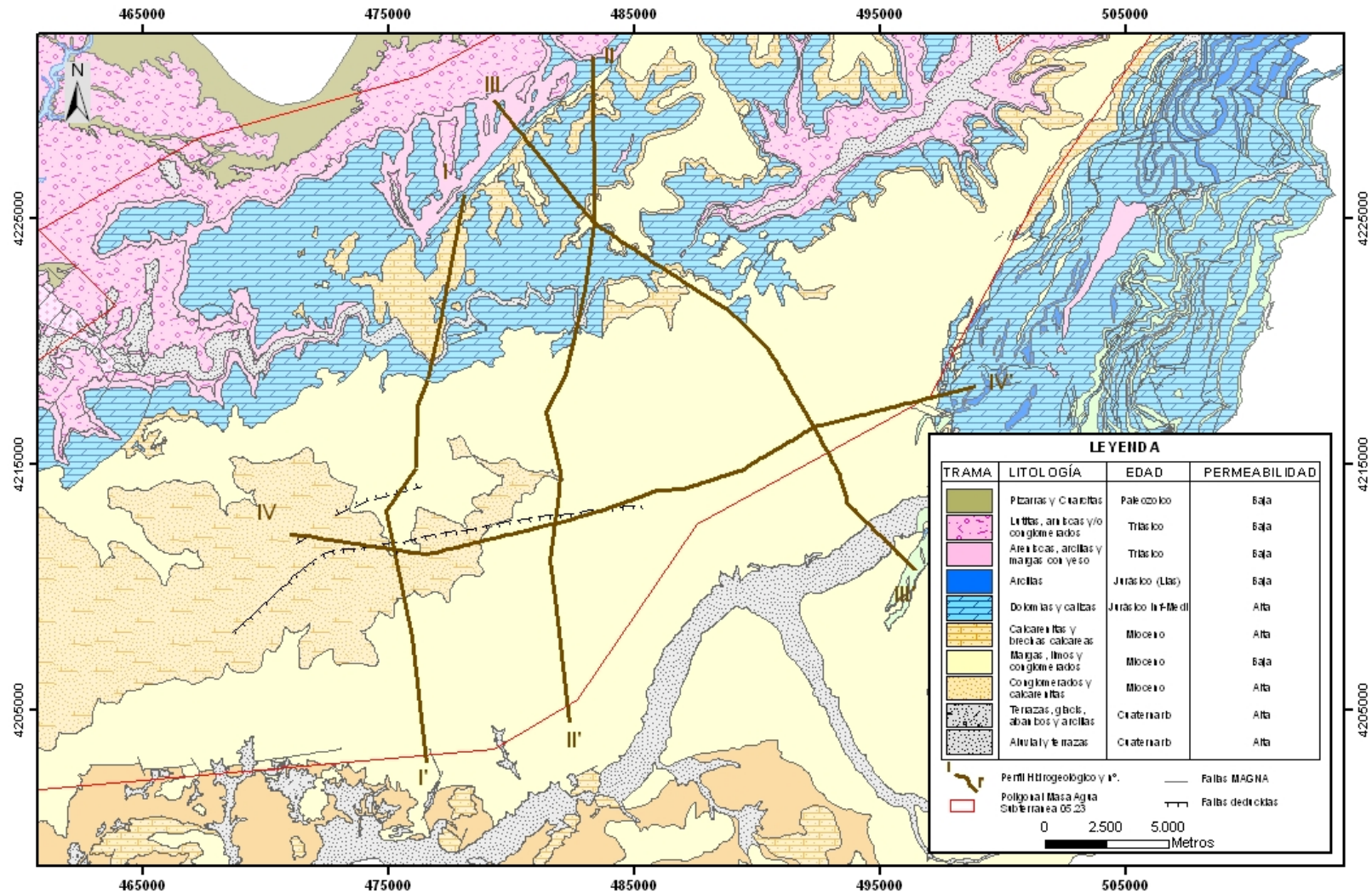
Figura 2.- Esquema geológico y situación de perfiles hidrogeológicos.
