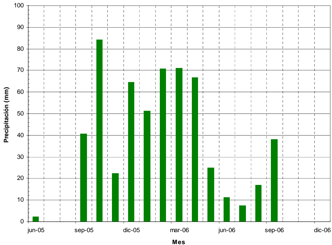
FIGURA 6 b.- Precipitaciones en la estación de Castellar de Santistéban
