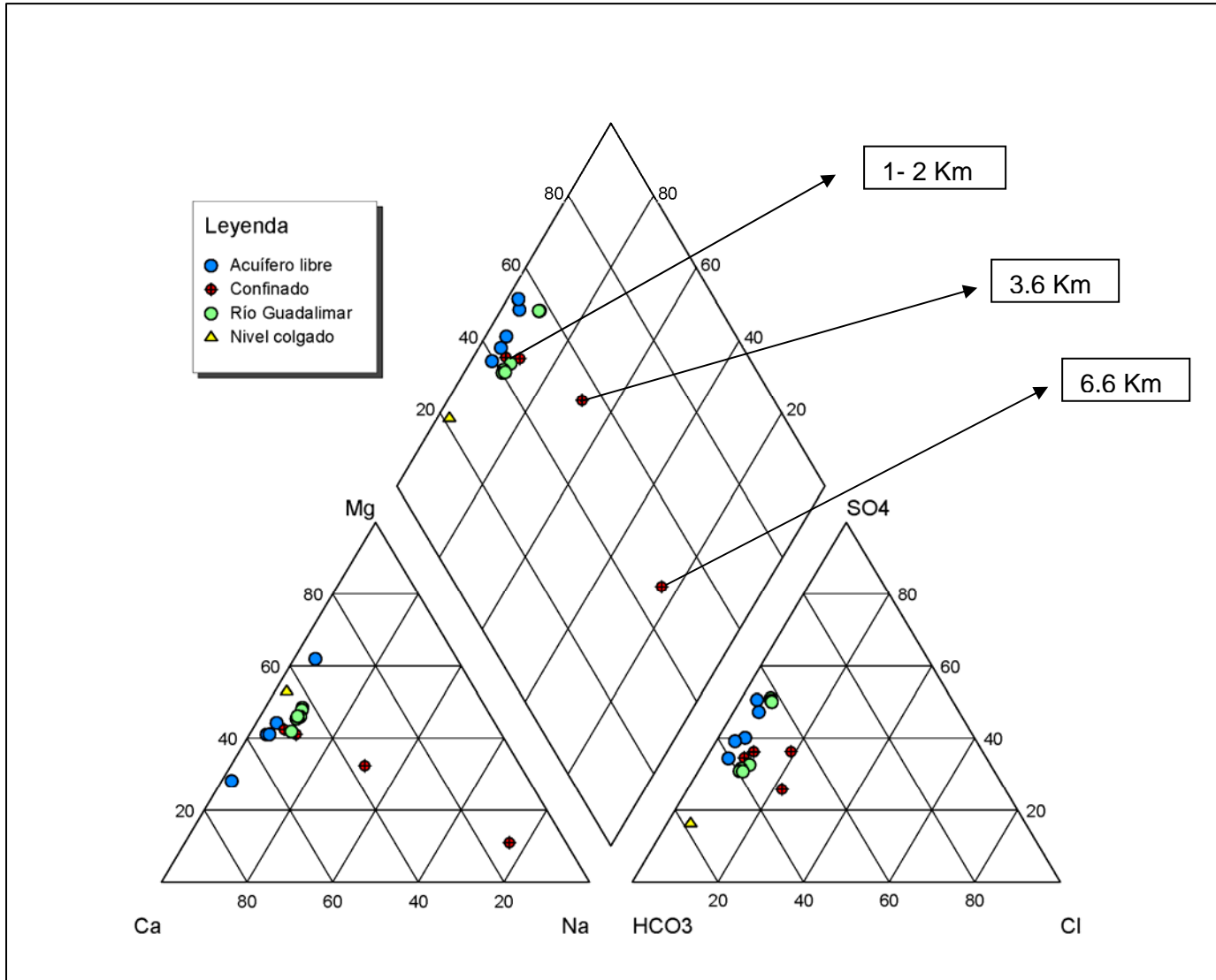
Figura 17.- Diagrama de Piper del entorno del río Guadalimar
