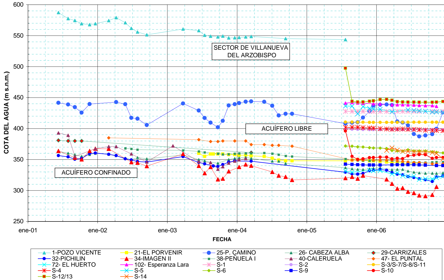
FIGURA 5.- ACUÍFERO CARBONATADO DE ÚBEDA. EVOLUCIÓN PIEZOMÉTRICA 2001-2006 (Acuífero confinado, libre y sector de Villanueva del Arzobispo)
