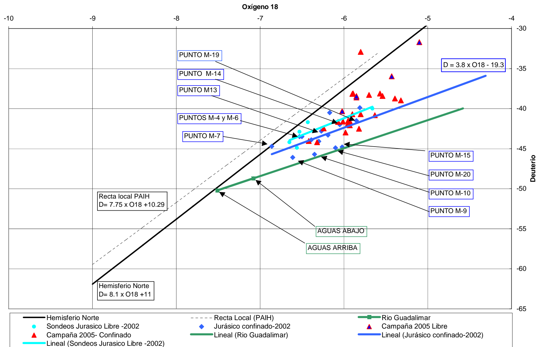
FIGURA 19.- Relación Deuterio-O18 (Muestreo CEDEX 2002 y Campaña IGME 2005)
