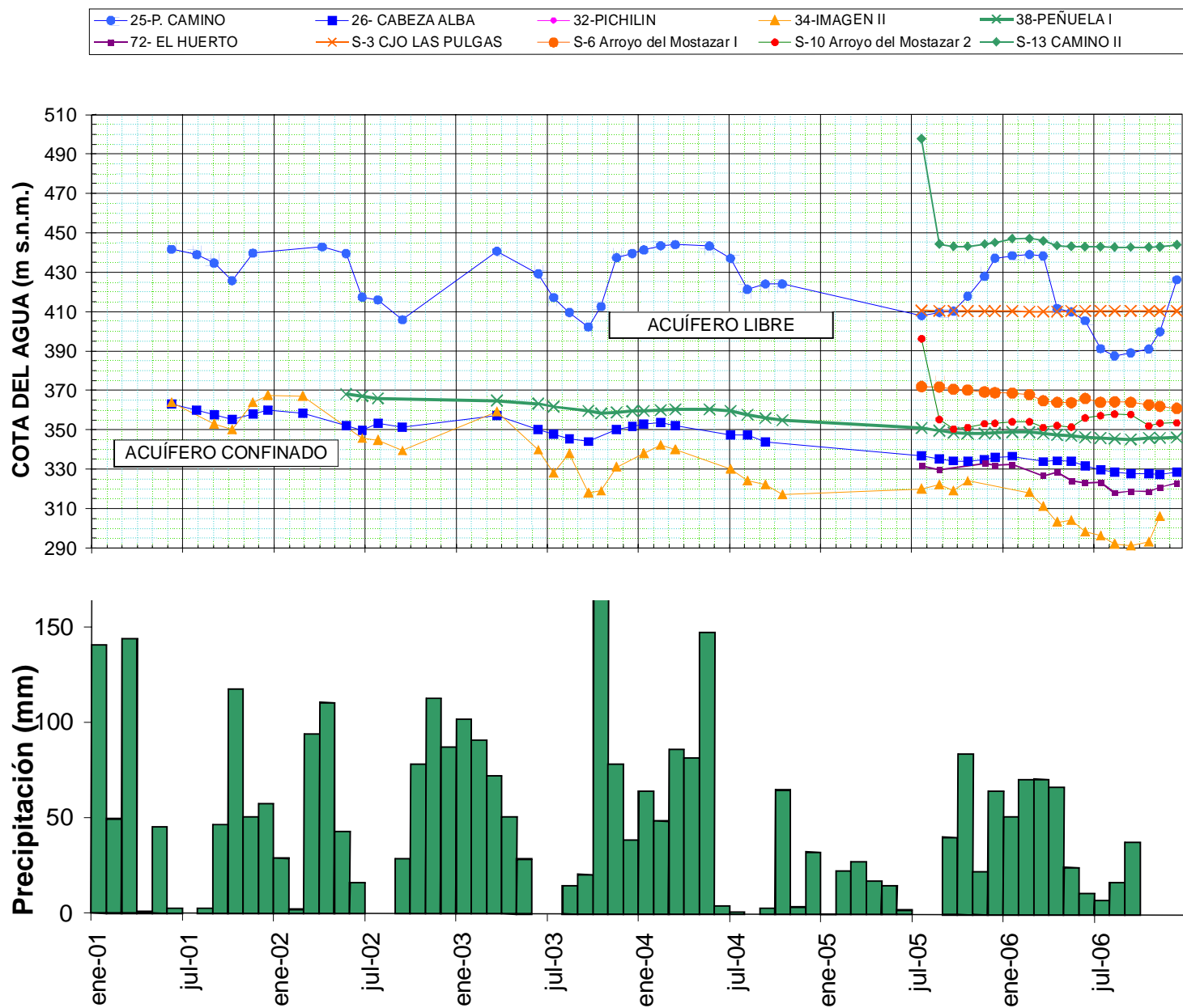
FIGURA 8.- ACUÍFERO CARBONATADO DE UBEDA. EVOLUCION PIEZOMETRICA 2001-2006 (Sondeos más representativos de la Red de Control)
